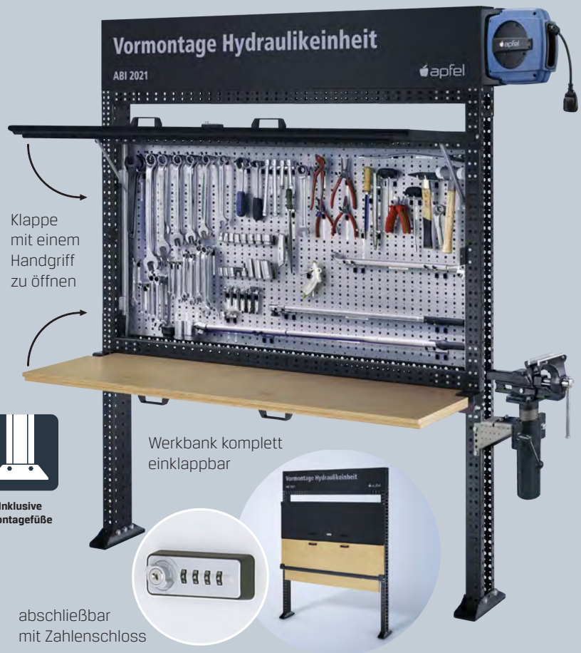
Werkbank einklappbar
